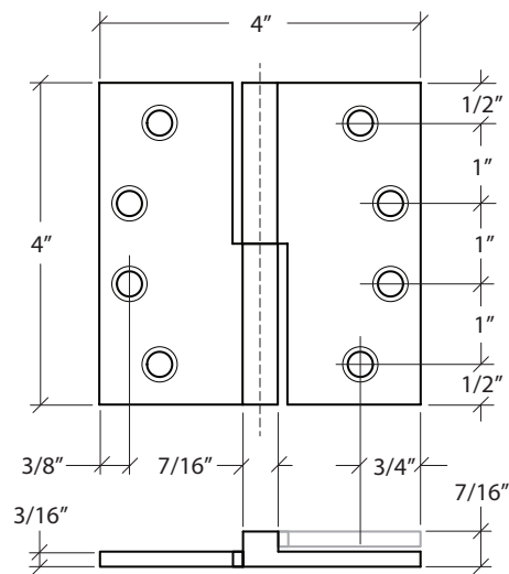
LEFT HAND HINGE SHOWN
